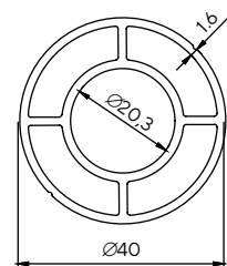
1099 0.956 kg/m
