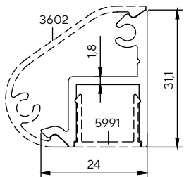
3601 0.388 kg/m
