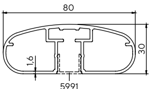
3604 1.146 kg/m
