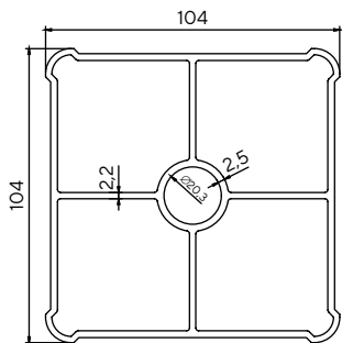
6700 3.891 kg/m
