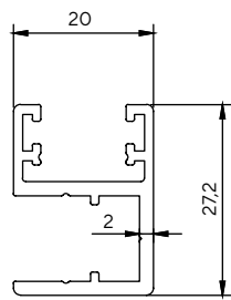
4097 0.420 kg/m
