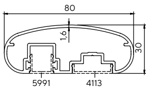
3605 1.123 kg/m
