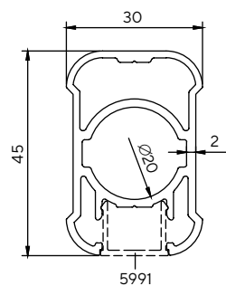
3603 0.987 kg/m
