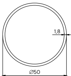
2984 0.738 kg/m
