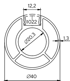
2246 0.855 kg/m
