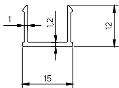
5991 0.108 kg/m
