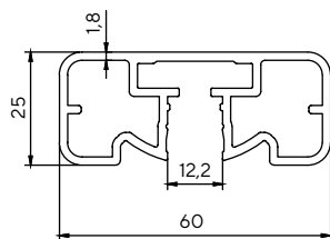
3628 1.109 kg/m
