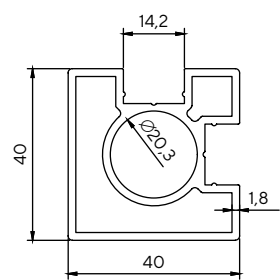
4699 1.156 kg/m
