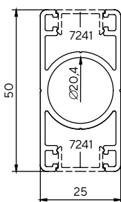
7252 0.857 kg/m
