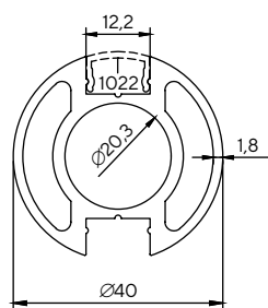
1010 1.143 kg/m
