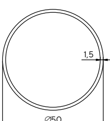
2622 0.620 kg/m
