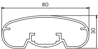
6688 1.058 kg/m
