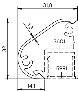
3602 0.275 kg/m
