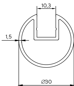
1570 0.467 kg/m
