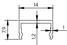
1411 0.080 kg/m
