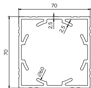
4117 2.437 kg/m
