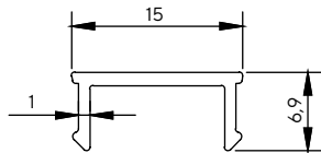
5992 0.080 kg/m
