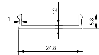
4113 0.108 kg/m
