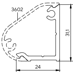
3618 0.357 kg/m
