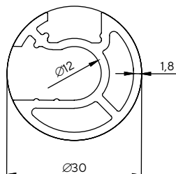
2825 0.598 kg/m
