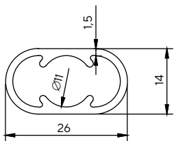
3609 0.316 kg/m
