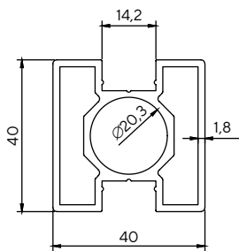
1410 1.188 kg/m
