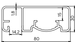
3629 1.271 kg/m
