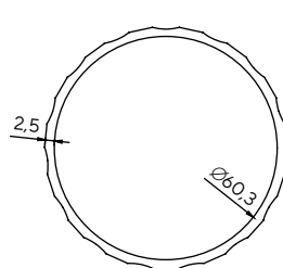
6023 1.266 kg/m
