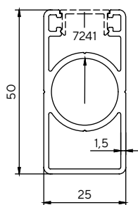
7253 0.872 kg/m
