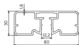
3630 1.397 kg/m
